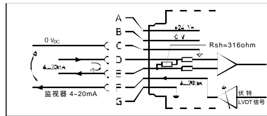
图D 误差输入信号
