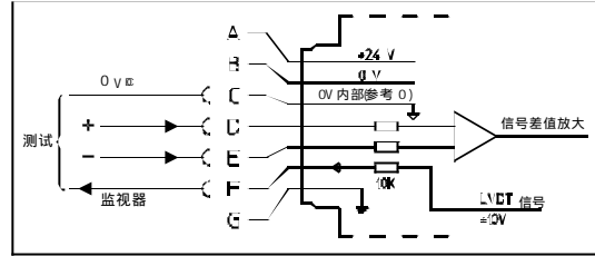
图B 误差信号不接地(浮动连接)
