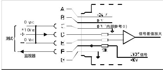
图A 电源和信号共零
